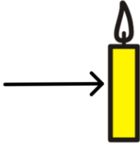
WOSK
