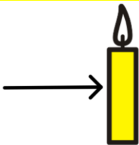
WOSK
